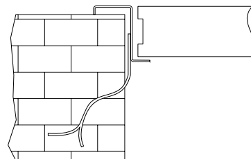
Telaio a "Z" a murare
