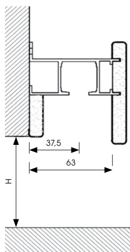
SEZIONE VERTICALE
