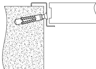
Telaio con guarnizione a tassellare
