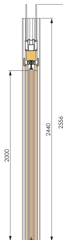
SEZIONE VERTICALE VERTICAL SECTION
