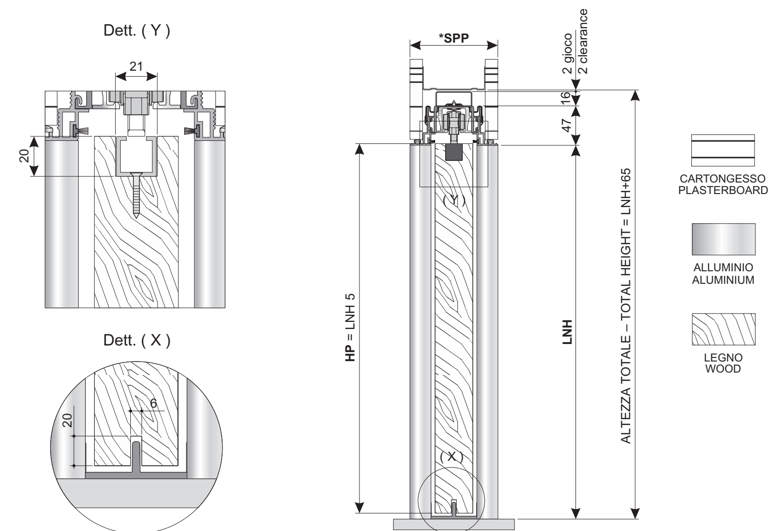
SEZIONE LONGITUDINALE - LONGITUDINAL SECTION
